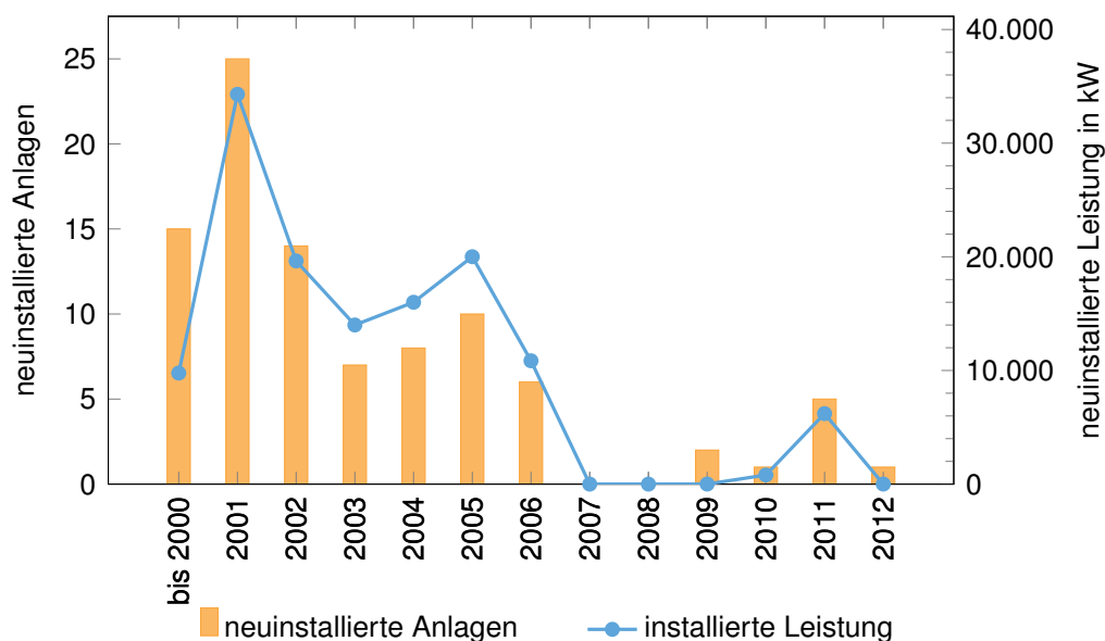
Abbildung 2.13: Installierte Windkraftanlagen und installierte Leistung pro Jahr
