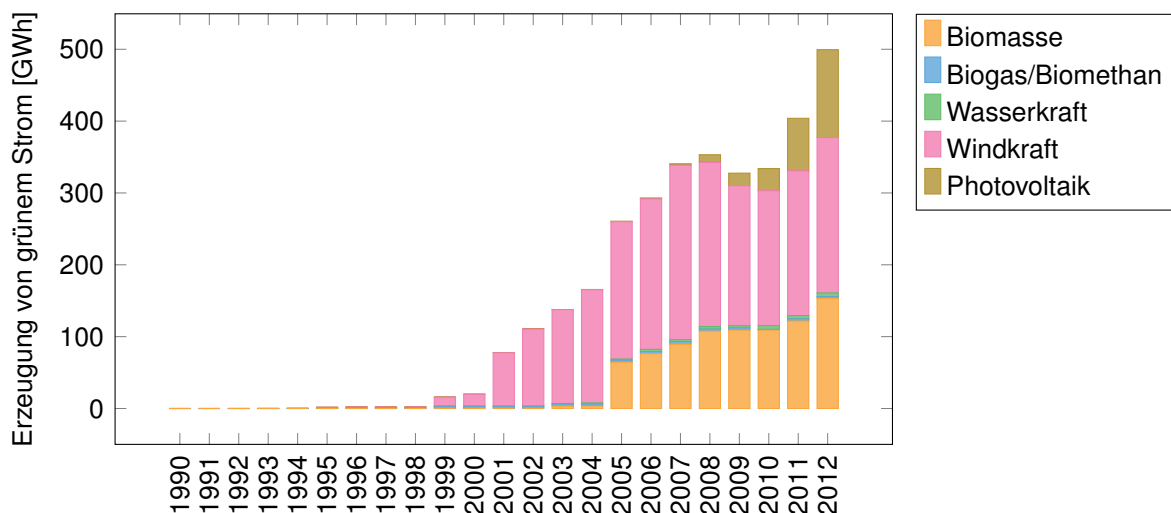
Abbildung 2.7: Jährliche Gesamtproduktion von „Grünem Strom“ im Landkreis Bautzen, unterteilt nach erneuerbaren Energiequellen
