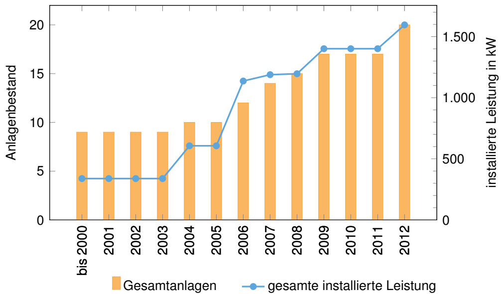
Abbildung 2.18: Wasserkraftanlagenbestand und installierte Leistung
