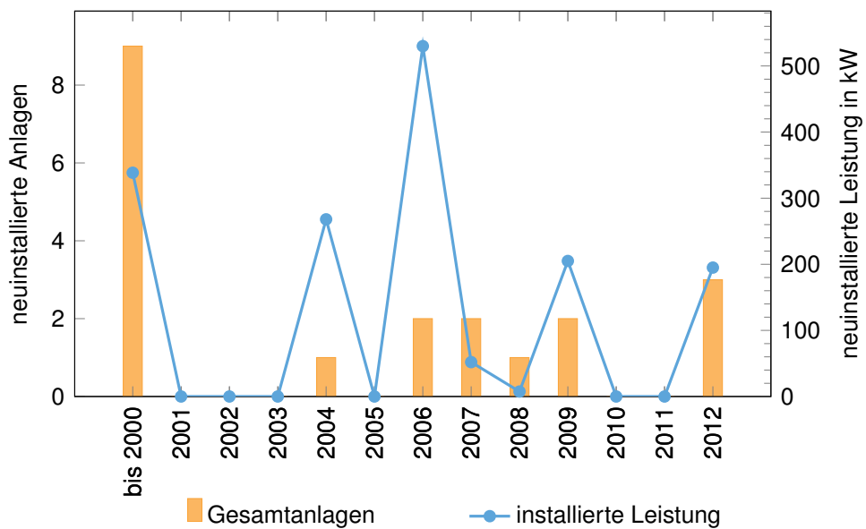
Abbildung 2.19: Installierte Wasserkraftanlagen und installierte Leistung pro Jahr
