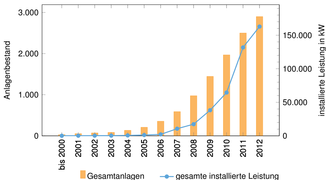
Abbildung 2.14: Photovoltaikanlagenbestand und installierte Leistung bis 2012
