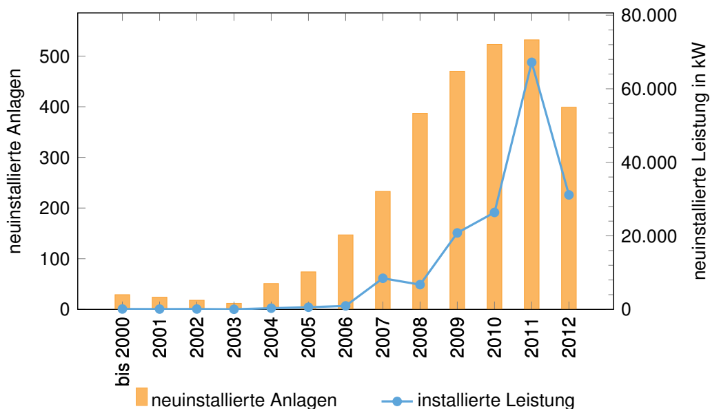
Abbildung 2.15: Installierte Photovoltaikanlagen und installierte Leistung pro Jahr
