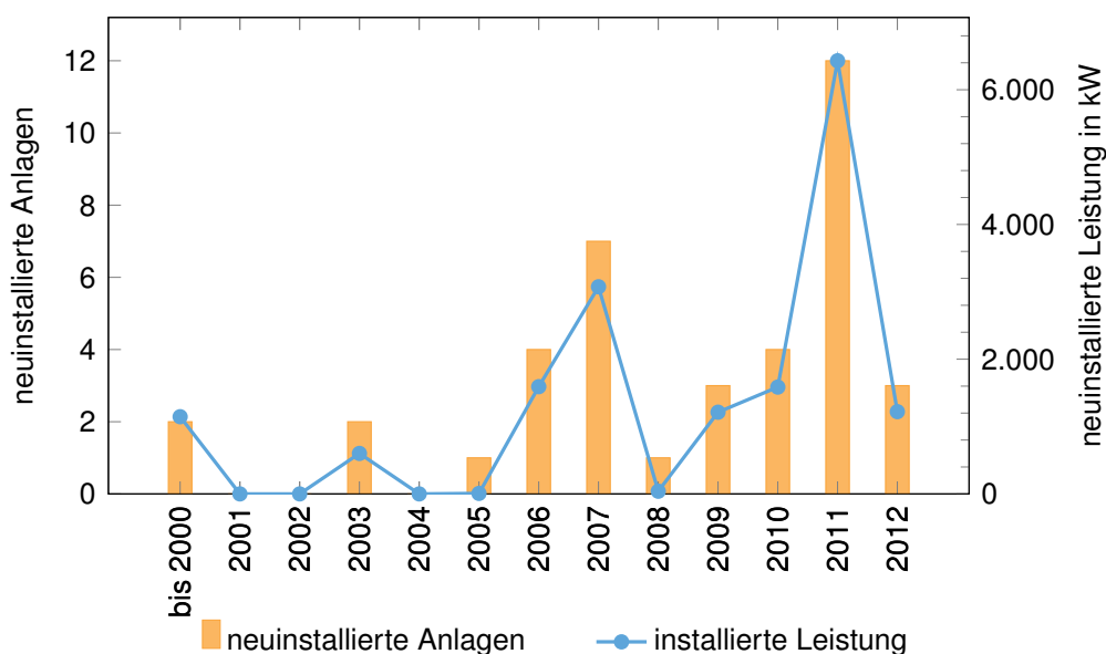
Abbildung 2.17: Installierte Biogas-/Biomasseanlagen und installierte Leistung pro Jahr
