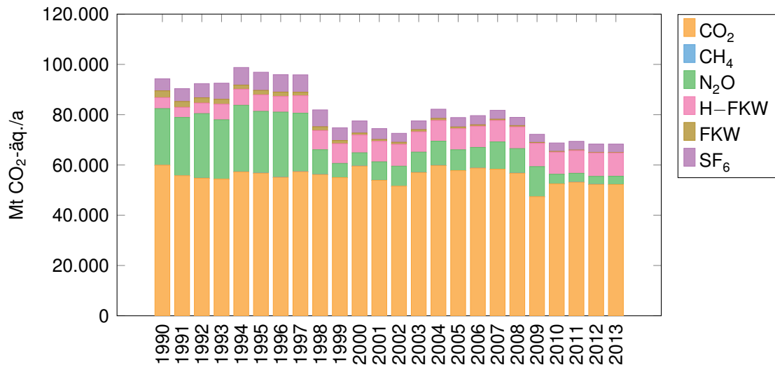
Abbildung 2.22: THG-Emissionen aus industriellen Prozessen (UBA, 2013c)
