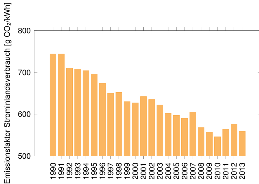
Abbildung 2.2: Entwicklung der Emissionsfaktoren im deutschen Strommix
