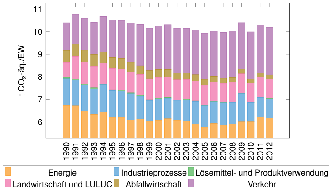
Abbildung 3.1: THG-Emissionen aller Sektoren pro Kopf für den Landkreis Bautzen
