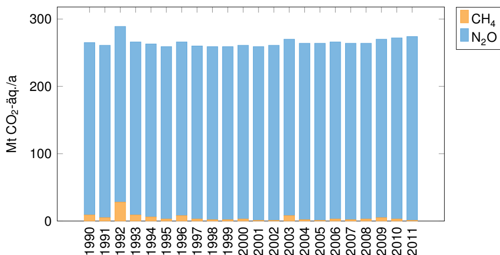
Abbildung 2.26: Landnutzung, Landnutzungsänderungen und Forstwirtschaft (UBA, 2013b)
