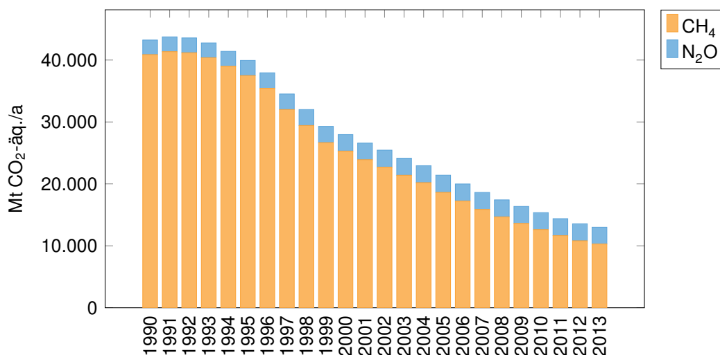
Abbildung 2.27: Entwicklung der gesamtdeutschen THG-Emissionen im Sektor Abfallwirtschaft
