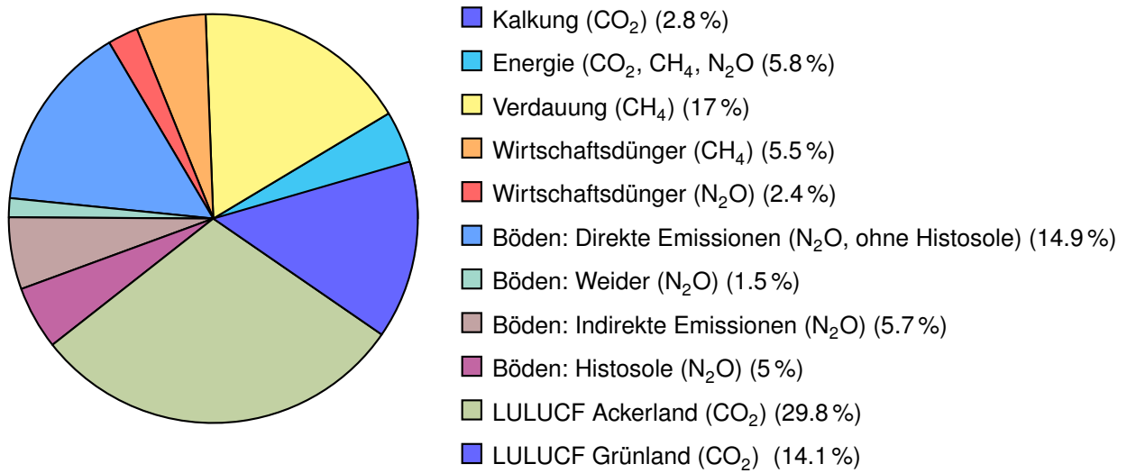
Abbildung 2.23: THG-Emissionen des deutschen Agrarsektors a
