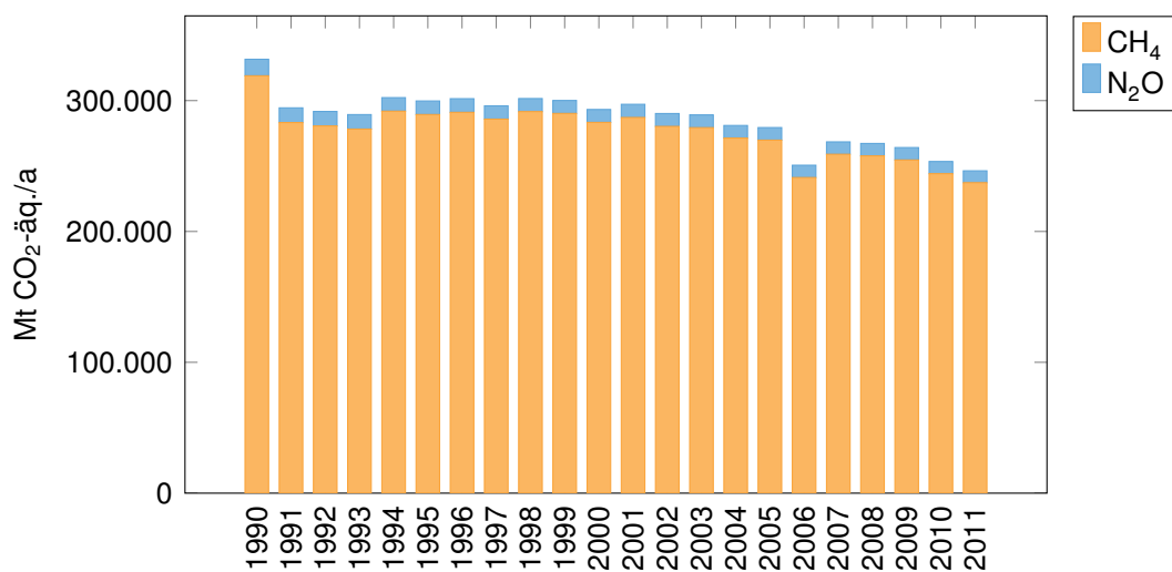
Abbildung 2.25: Emissionen aus Landwirtschaftlichen Böden (UBA, 2013b)
