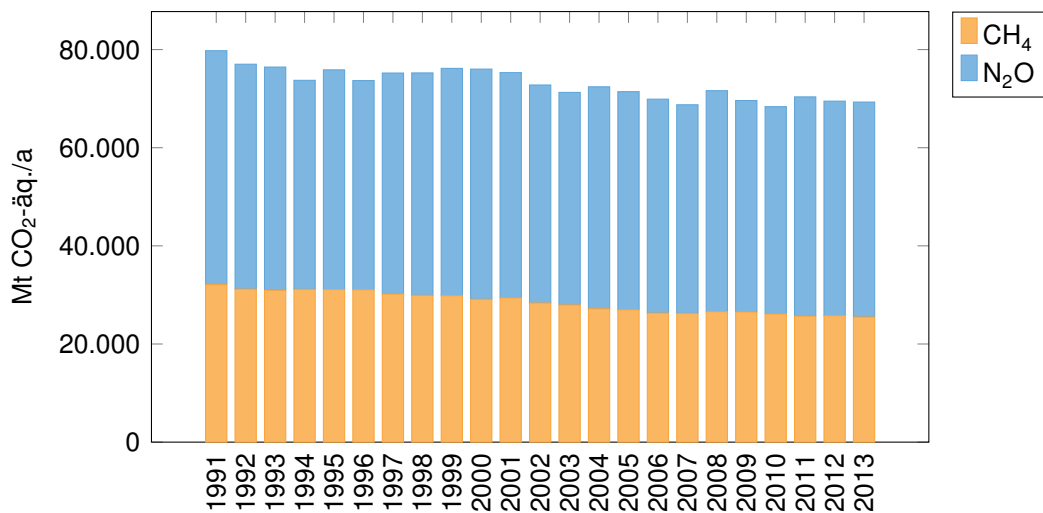
Abbildung 2.24: Methan und Distickstoffoxid-Emissionen aus dem Sektor Landwirtschaft (UBA, 2013b)
