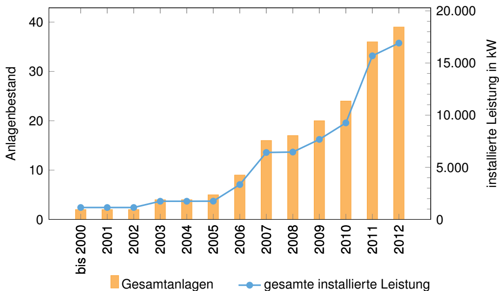
Abbildung 2.16: Biomasse-/Biogasanlagenbestand und installierte Leistung bis 2012
